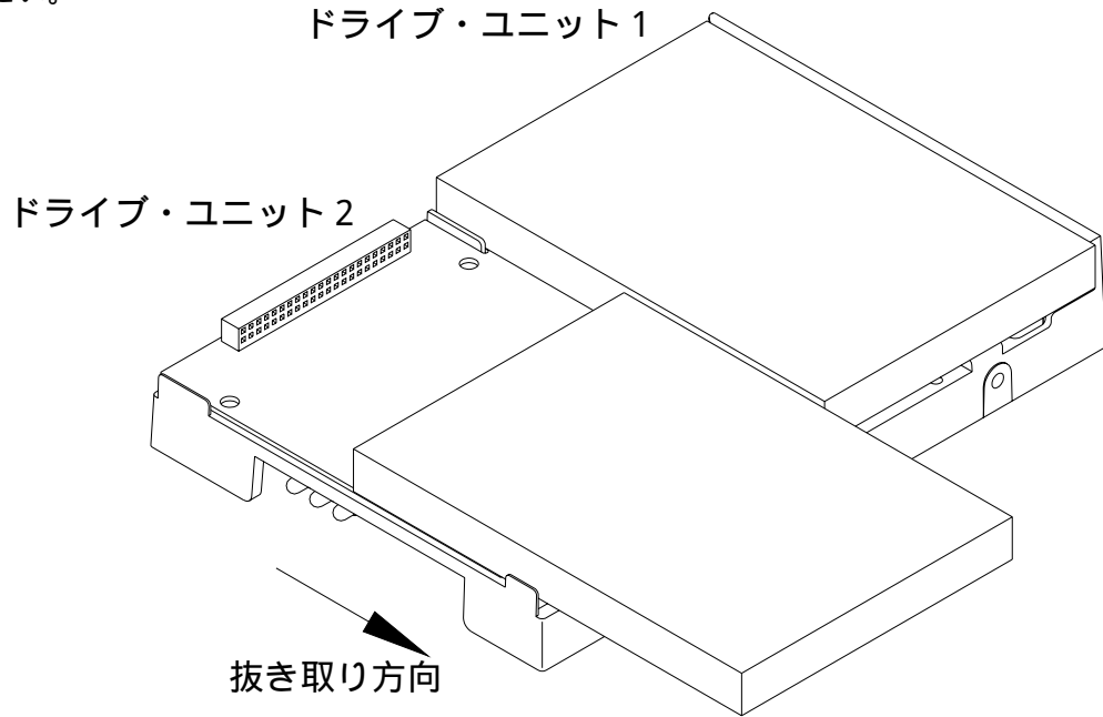
ドライブ・ユニットの抜き取り方向
