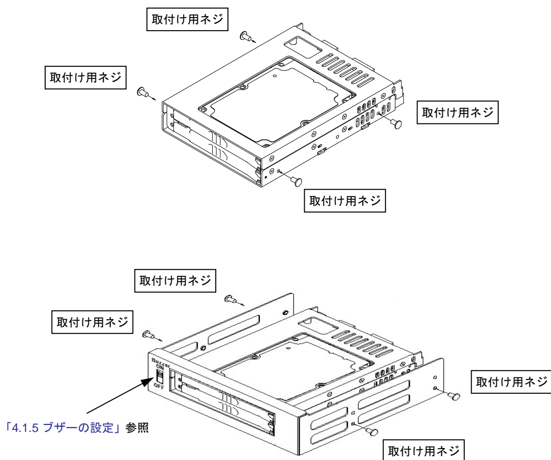
側面の取付け用ネジ穴を使用した場合
